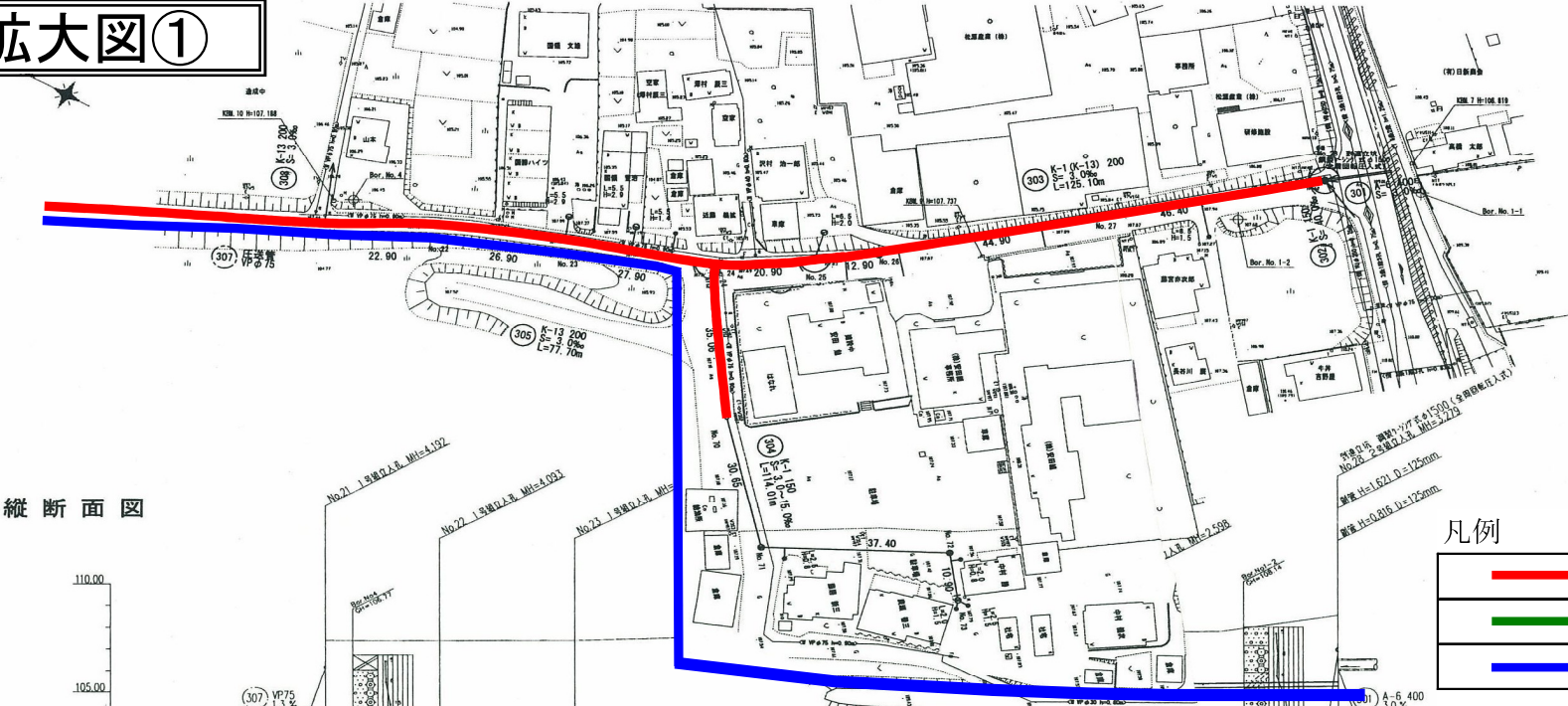
1-A1-1 詳細図
