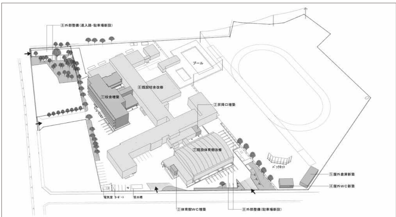
愛知川東小学校改築工事(全体配置イメージ図)
