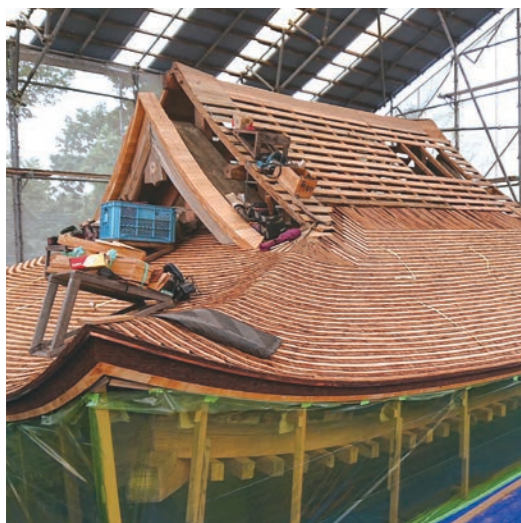
屋根を葺替えている四脚門(令和3年9月)
