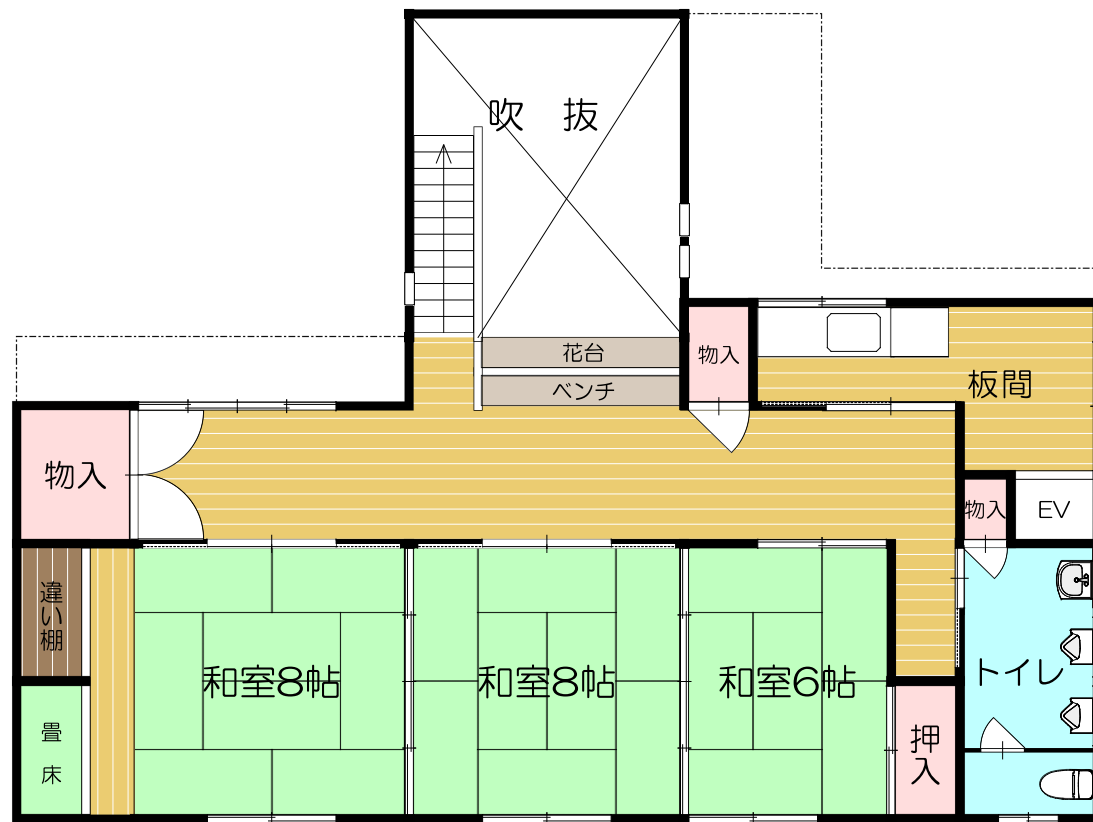
2階平面図
