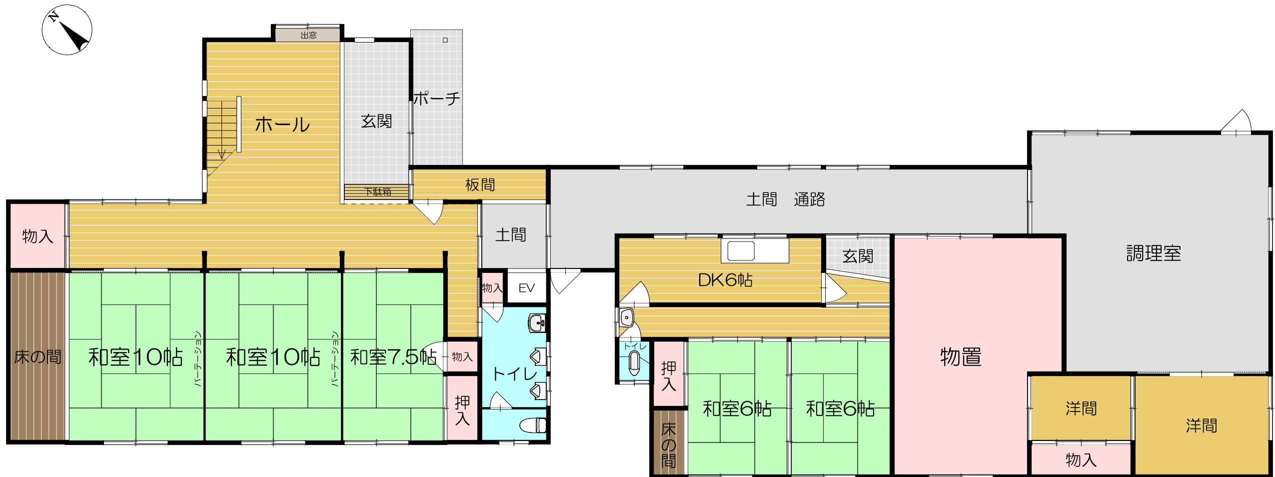
1階平面図
