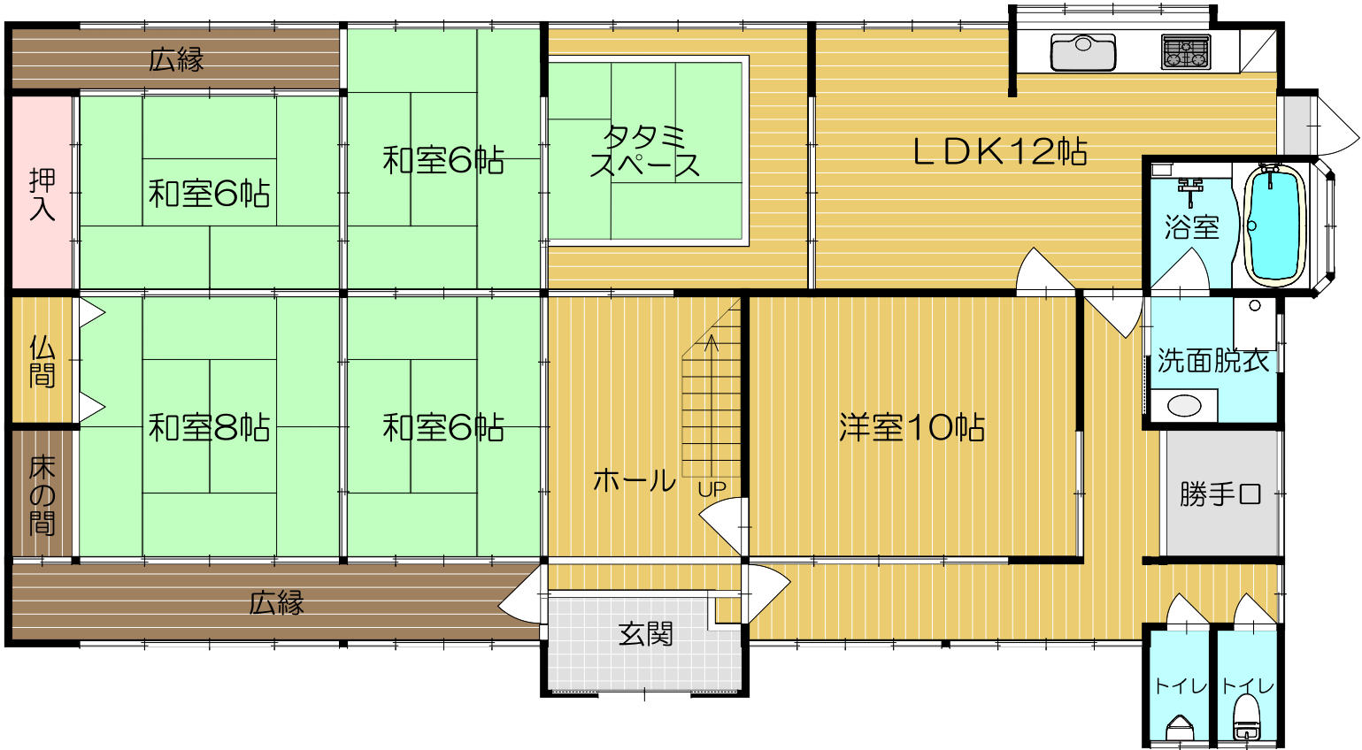
1階平面図
