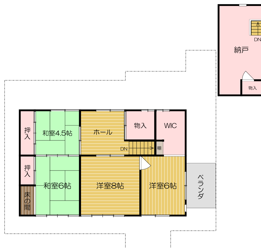
2階平面図
