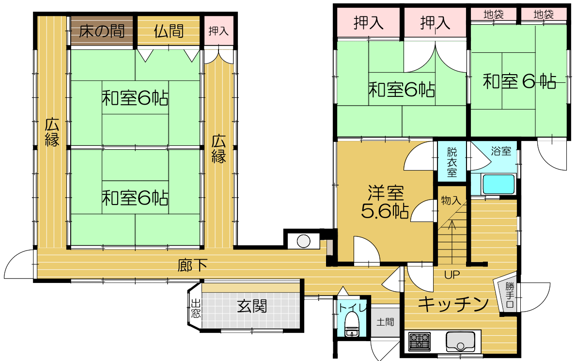
1階平面図
